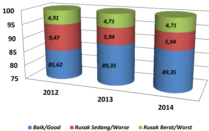
Gambar 11. Kondisi Jalan di Jayapura , Tahun 2012-2014
